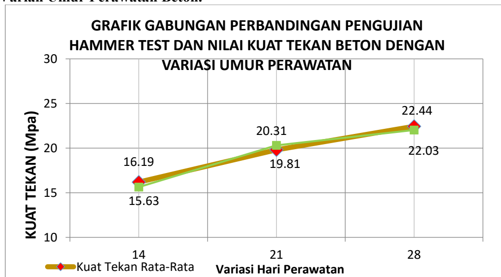
Gambar 4. Grafik Perbandingan Pengujian Hammer Test dan Kuat Tekan Beton Dengan Variasi Hari Perawatan
